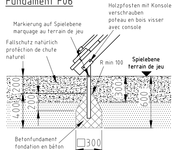
Fundament F06
