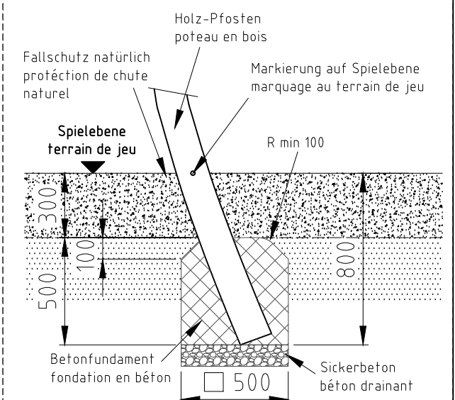
Fundament F31
