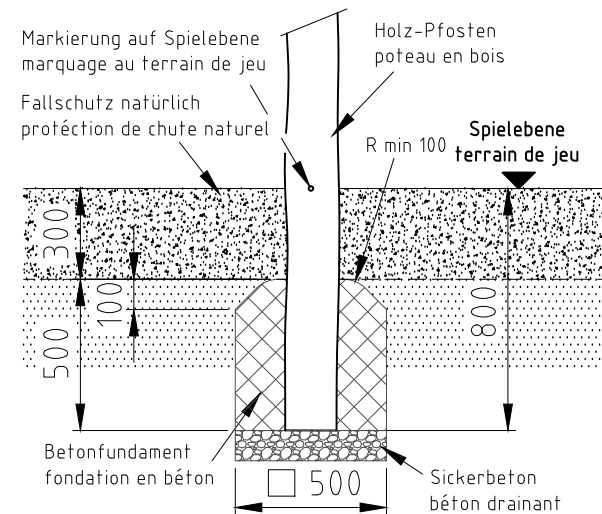
Fundament F06
